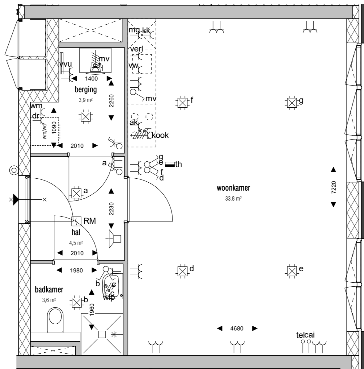
Woningtype S1B bnr: 468, 481 1 : 50
