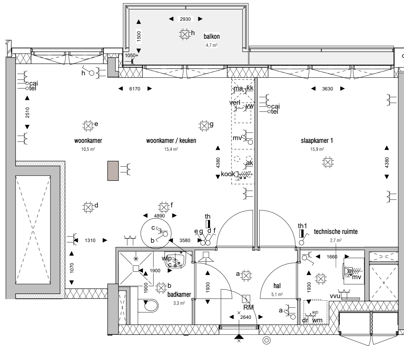
Woningtype R6F bnr: 462,475 1 : 50
