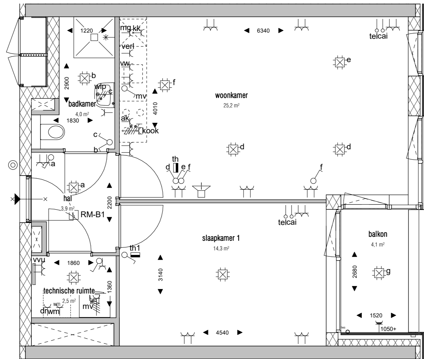
Woningtype R2D bnr: 310, 319, 328, 337 1 : 50
