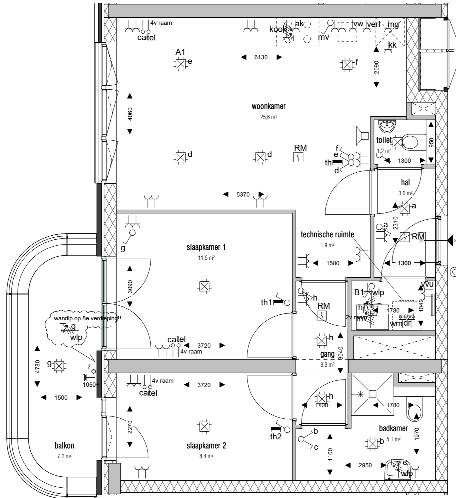
Woningtype R6A bnr: 316, 325, 334, 343, 350, 357, 364 1 : 50
