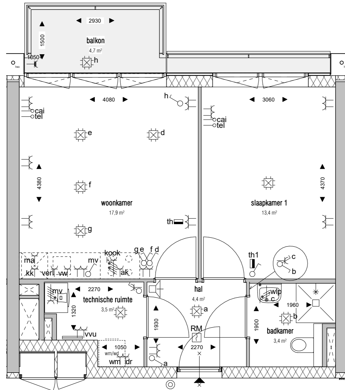
Woningtype R2H bnr: 464, 477 1 : 50
